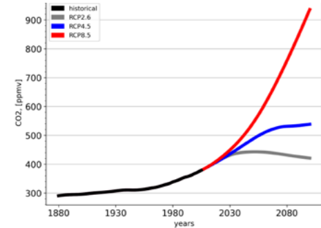
Abbildung 2: Historische und zukünftige jährliche atmosphärische CO 2 -Äquivalentkonzentrationen der RCP-Szenarien
