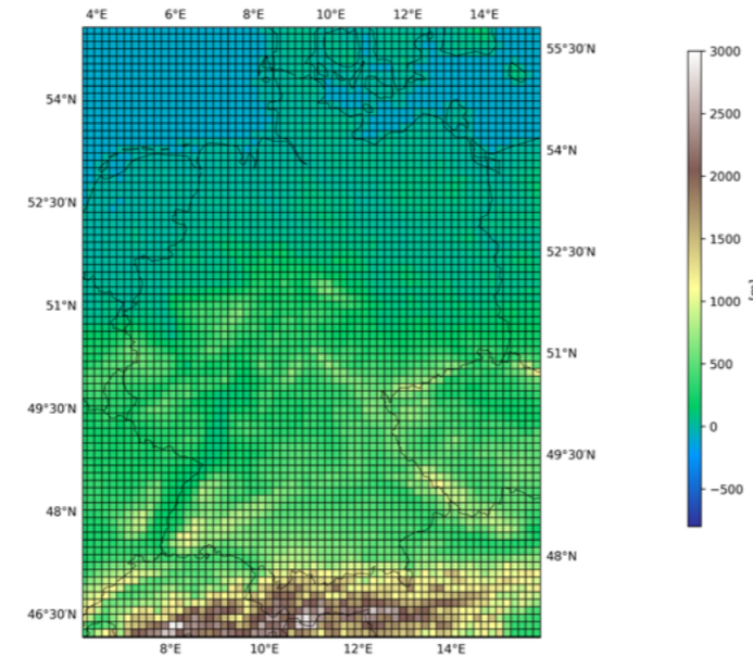
Abbildung 3: Schematische Darstellung der Modellgitter des Regionalklimamodells REMO. Die Auflösung der Atmosphäre beträgt 12 km. Die Beschriftungsleiste zeigt die Orographie des REMO.
