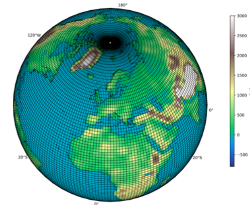
Abbildung 1: Schematische Darstellung der Modellgitter des ESM des Max-Planck-Instituts für Meteorologie (MPI-ESM-LR). Die Auflösung der Atmosphäre beträgt 1,8°. Die Beschriftungsleiste zeigt die Orographie des ESM.
