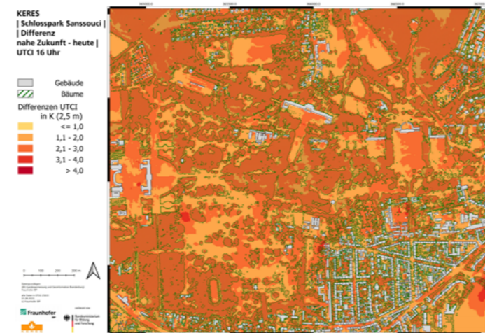
Abbildung 10: Darstellung der Veränderung der Hitzebelastung Mitte des 21. Jahrhunderts (2036-2065), ausgehend vom heutigen Stand. In sämtlichen Bereichen ist mit einer erhöhten Hitzebelastung zu rechnen, auch an baumbestandenen Standorten erhöht sich die Belastung um bis zu 3 °C. © Fraunhofer IBP
